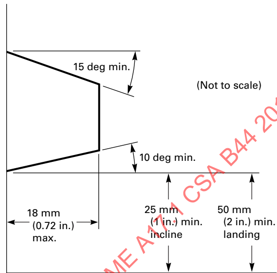
Fig. 6.1.3.3.10 Dimensions
