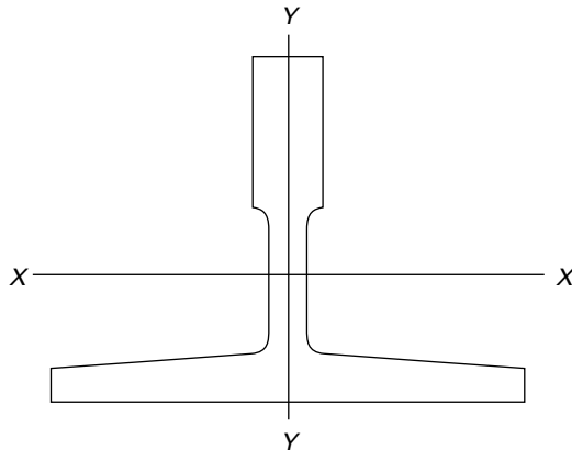
Fig. 8.4.8.9 Guide-Rail Axes
