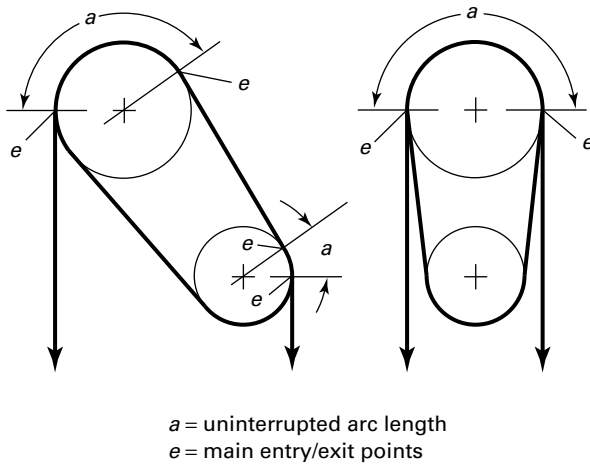
Fig. 8.4.3.1.3 Arc of Contact
