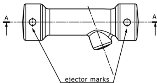
FIG. X2.3 Ejector Marks
