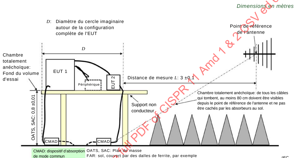
Figure 3b – Vue de côté
