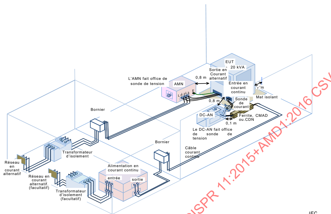
Figure 9 – Configuration classique pour le mesurage des perturbations conduites aux accès d'alimentation en courant continu à basse tension, un DC-AN étant utilisé comme sonde de tension et avec une sonde de courant – schéma 3D
