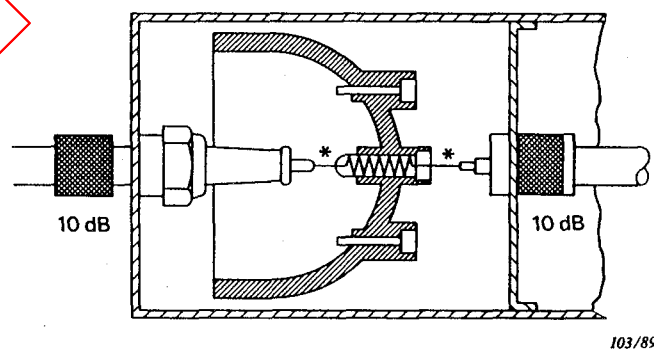
Figure E.8 — Balai résistant dans la tête du distributeur
