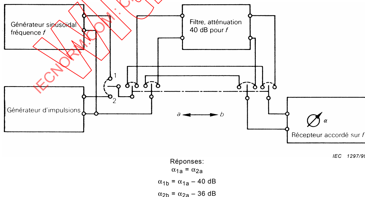
Figure 3 – Schéma pour l'essai des effets d'intermodulation
