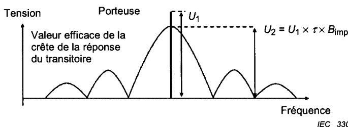
Figure E.6 – Filtrage avec une B_{imp} nettement plus large que la prf
