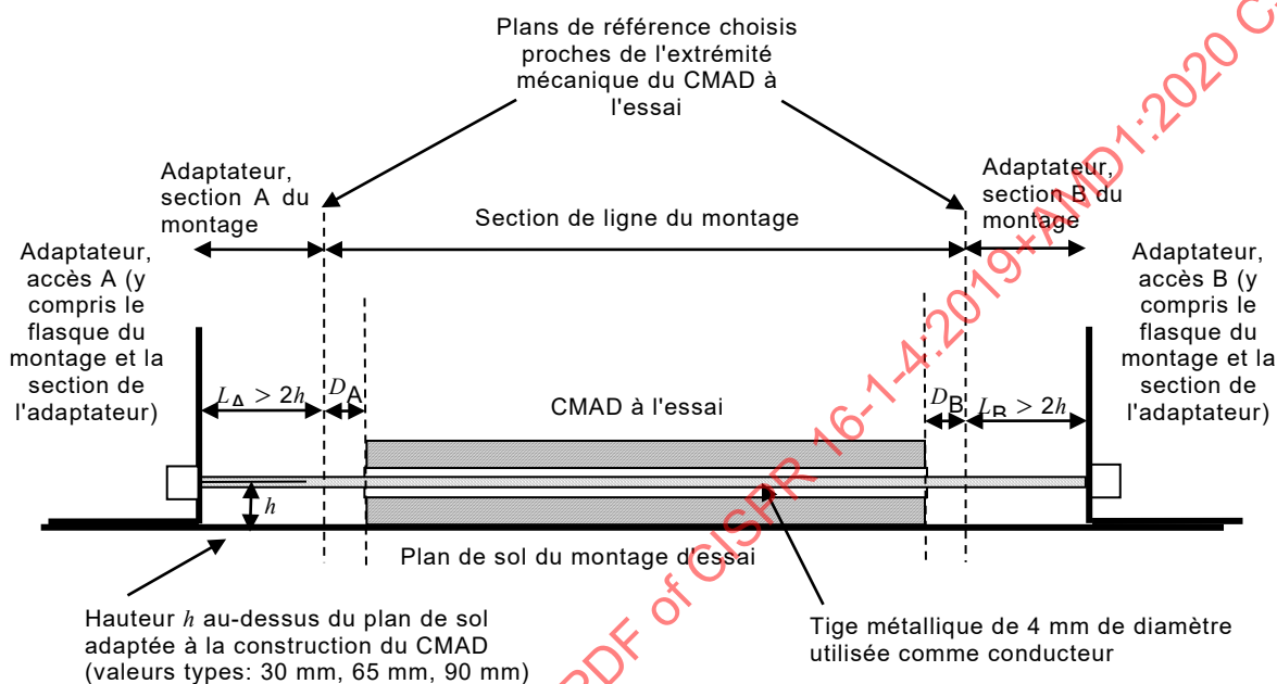
Figure 26 – Définition des plans de référence à l'intérieur du montage d'essai
