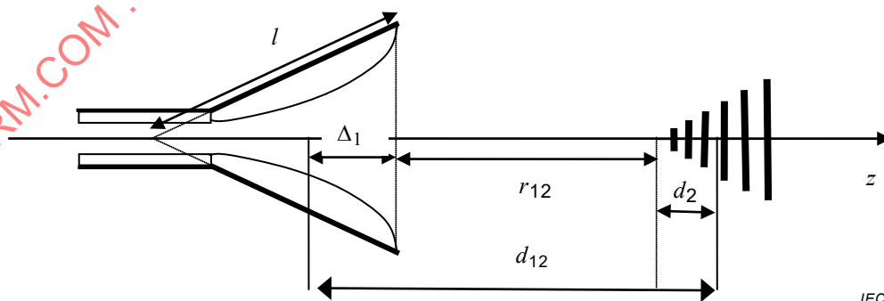
Figure D.1 – Centres de phase relatifs d'une antenne DRH et d'une antenne LPDA
