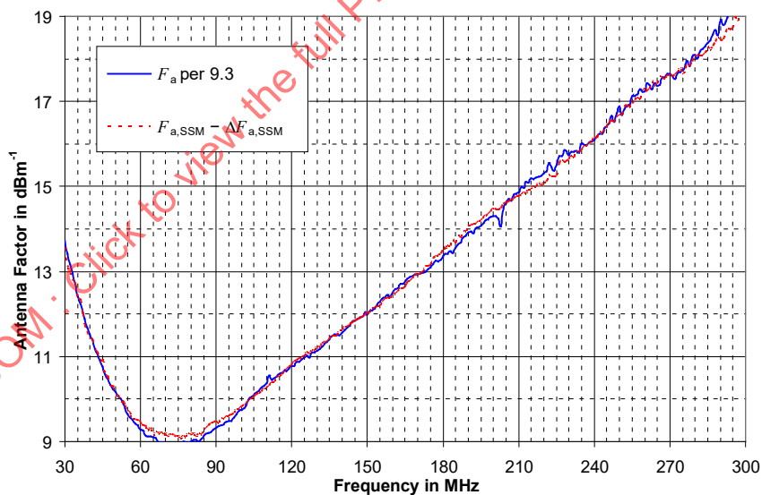
Figure A.2 – Facteur F_a d'une antenne biconique avec un symétriseur de 200 \Omega , mesuré par la méthode VP de 9.3 et par la méthode SSM de 8.4 sans correction
