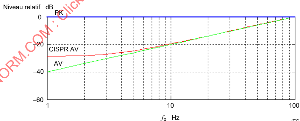
Figure D.2 – Fonctions de pondération d'une impulsion de 10 ms pour des détections de valeurs de crête ("PK") et moyennes avec ("CISPR AV") ou sans ("AV") relevé de crête; avec un contrôleur de période de 100 ms
