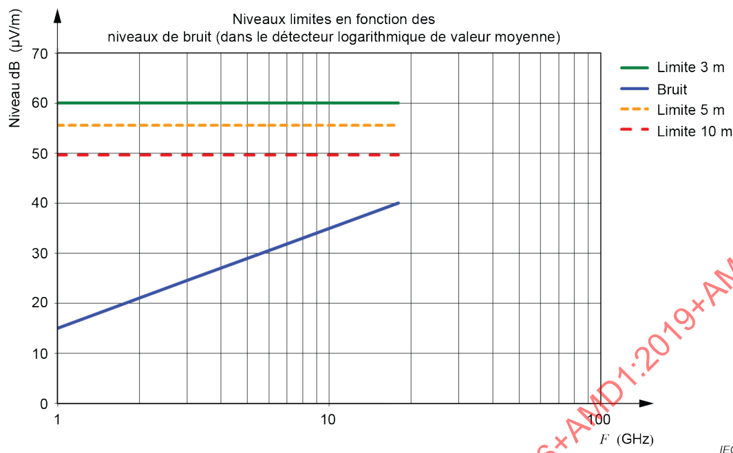
Figure F.8 – Niveau de bruit E_{\text{Nlogav}} (exemple pour 10 \lg F_{\text{tot}} = 4 \text{ dB} ) comparé à la limite de perturbation E_{\text{Lav}} pour le détecteur logarithmique de valeur moyenne pour des distances de 3 m, 5 m et 10 m dans la plage de fréquences comprises entre 1 GHz et 18 GHz
