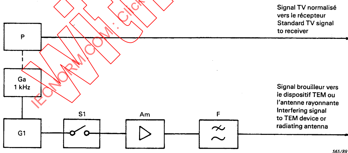
Figure 8 – Circuit de mesure pour l'immunité aux champs ambiants de téléviseurs (voir 5.2.3.2)
