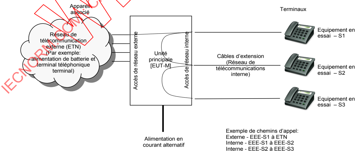
Figure A.5 – Exemple de système de téléphonie à auto-commutateurs privés classique ou PABX
