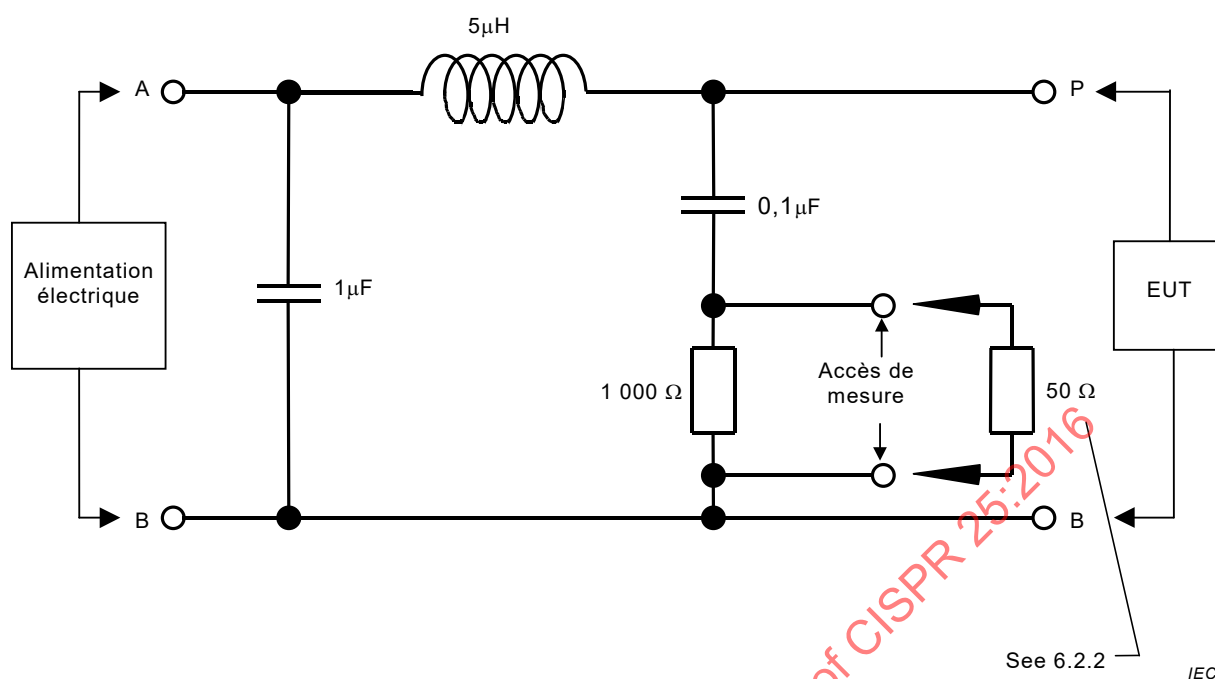
Figure E.1 – Exemple de schéma d'AN de 5 μH
