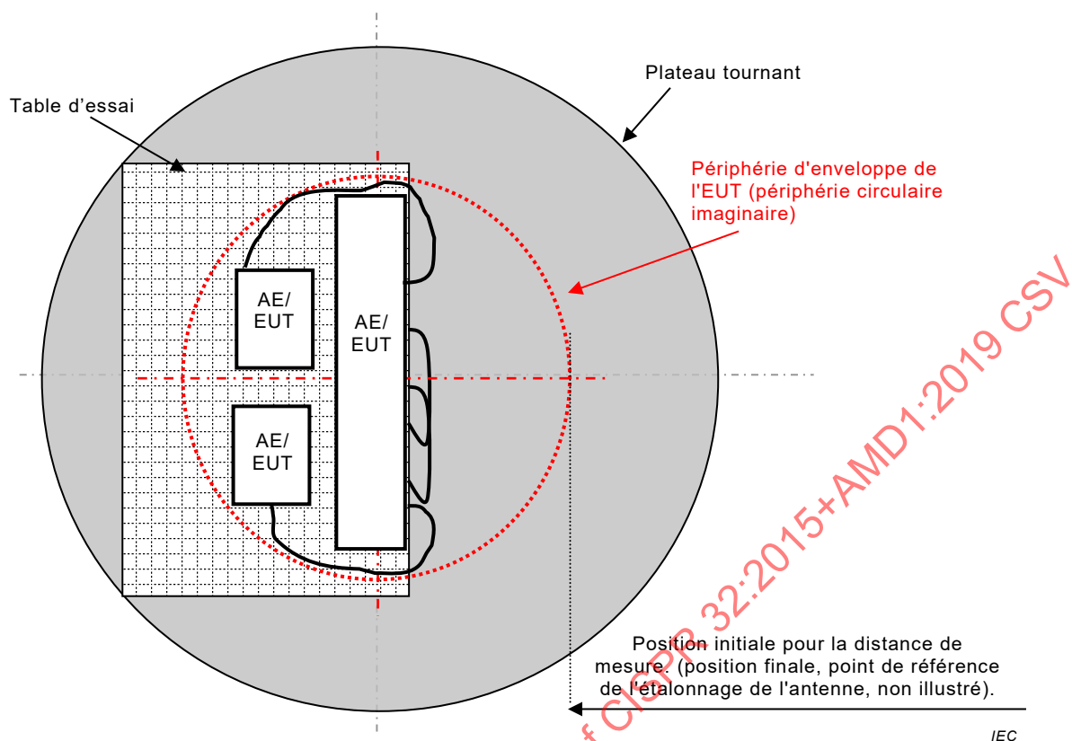
Figure C.2 – Périphérie d'enveloppe de l'EUT, de l'AE local et du câblage associé
