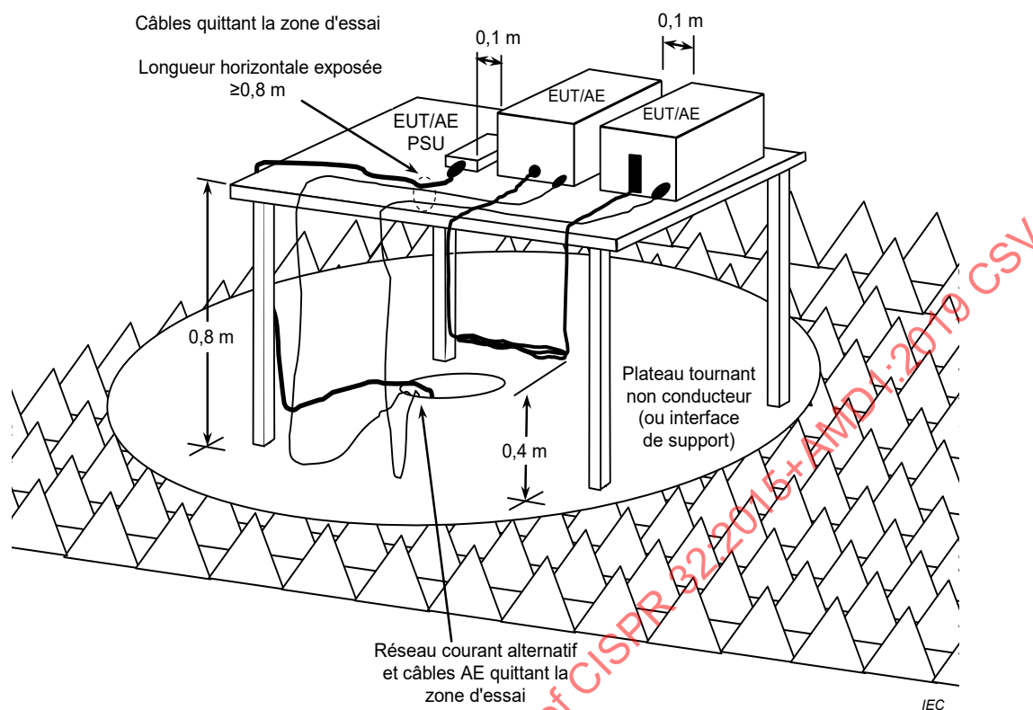
Figure D.11 – Exemple de disposition de la mesure pour l'EUT de dessus de table (mesure des émissions rayonnées dans une FAR)
