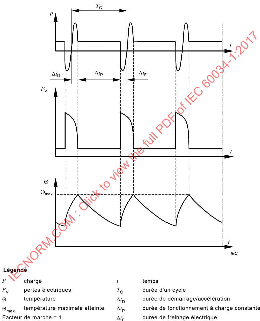
Figure 7 – Service ininterrompu périodique à freinage électrique – Service type S7
