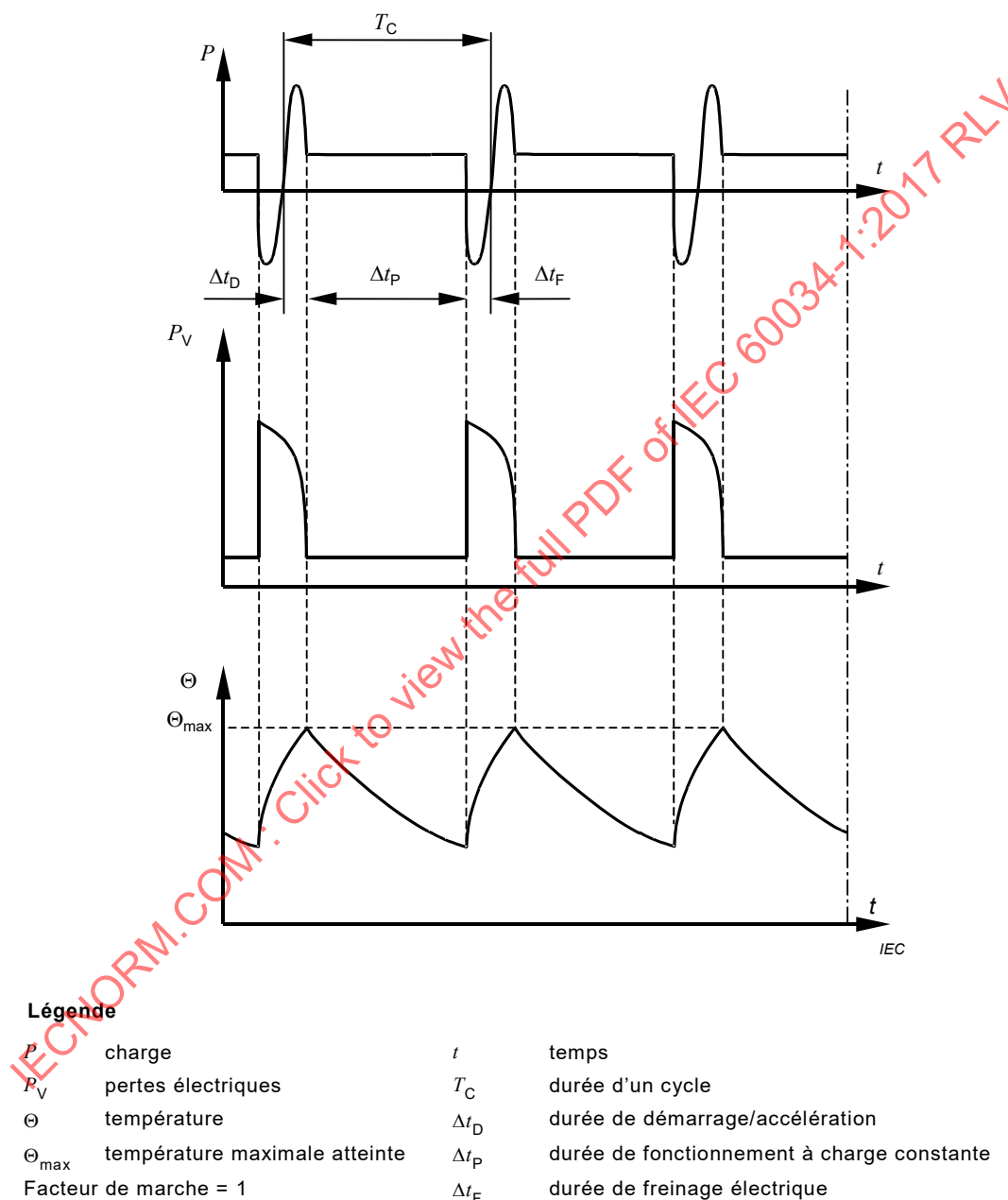
Figure 7 – Service ininterrompu périodique à freinage électrique – Service type S7
