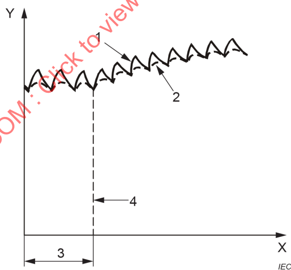
Figure 1 – Exemple de surcharge thermique à évolution lente et de protection thermique directe
