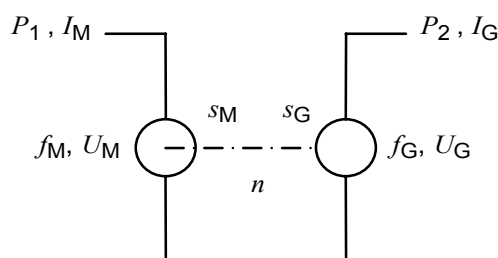
Figure 2 – Schéma pour l'essai en opposition à double alimentation (pour les machines synchrones: I_M = I_G, f_M = f_G )
