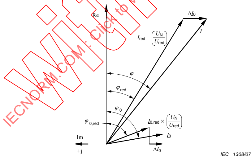
Figure 8 – Schéma vectoriel pour obtenir le vecteur courant à partir de l'essai à la tension réduite
