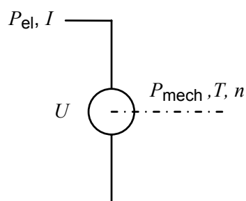
Figure 1 – Schéma pour l'essai de mesure du couple
