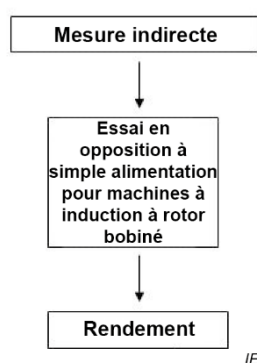
Figure 11 – Détermination du rendement selon la méthode 2-1-1E
