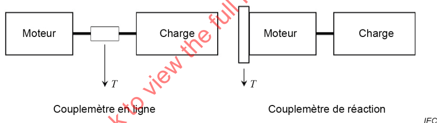
Figure 1 – Dispositifs de mesure de couple
