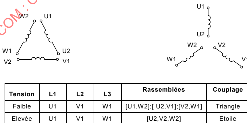
Figure A.3 – Deux tensions, six extrémités (1:√3)
