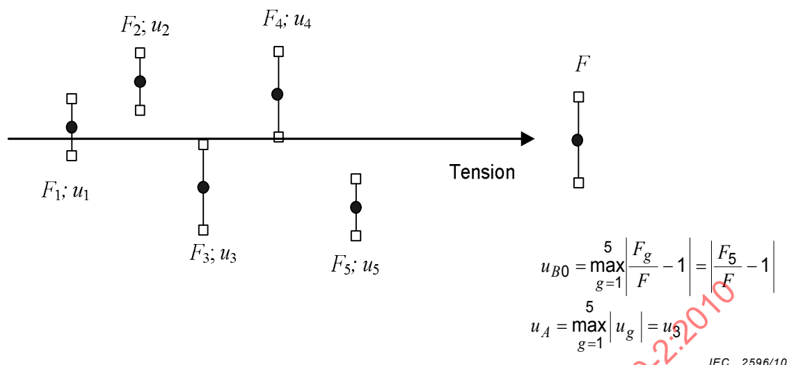
Figure 3 – Contributions d'incertitude de l'étalonnage (exemple avec un minimum de 5 niveaux de tension)
