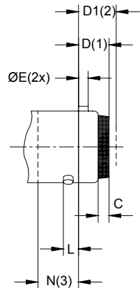
All other dimensions as for BAW15d Toutes les autres dimensions sont les mêmes que pour BAW15d
