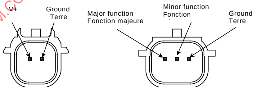
Figure 3 – Connector definition / Définition de connexion
