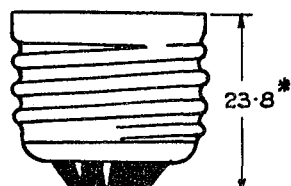
American standard domestic cap. Culot normal domestique américain
