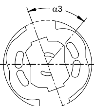
GX24q-5
