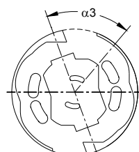
GX24q-6
