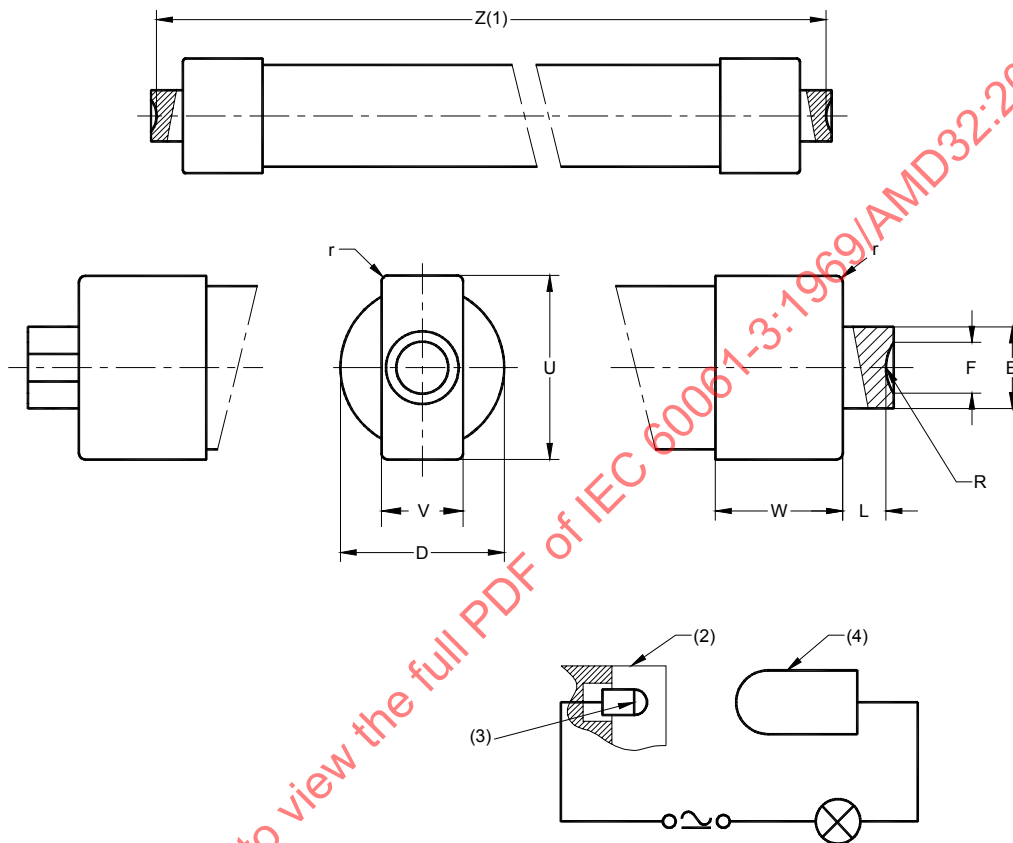
TEST CIRCUIT - CIRCUIT D'ESSAI
