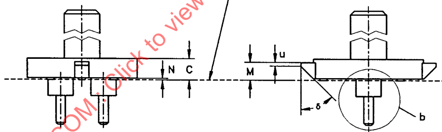
Reference plane Plan de référence
