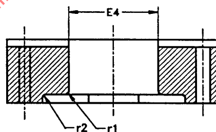
Section II-II Coupe II-II
