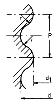
Detail of thread Détail du filetage
