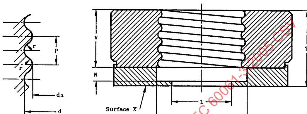
Detail of thread Détail du filetage
