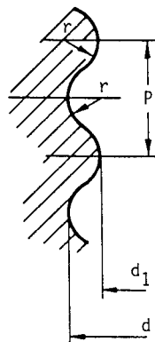
Detail of thread Détail du filetage
