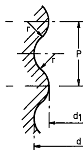
Detail of thread Détail du filetage
