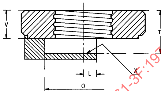
Right-hand thread Filet à droite
