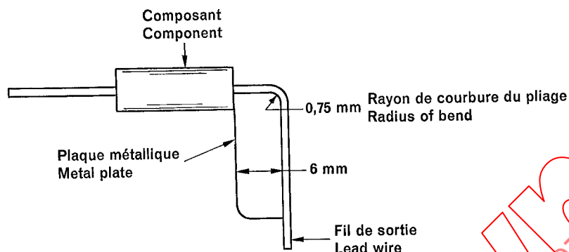
FIG 3a — Méthode de pliage du fil de sortie pour l'essai de torsion Method of bending wire leads for the torsion test
