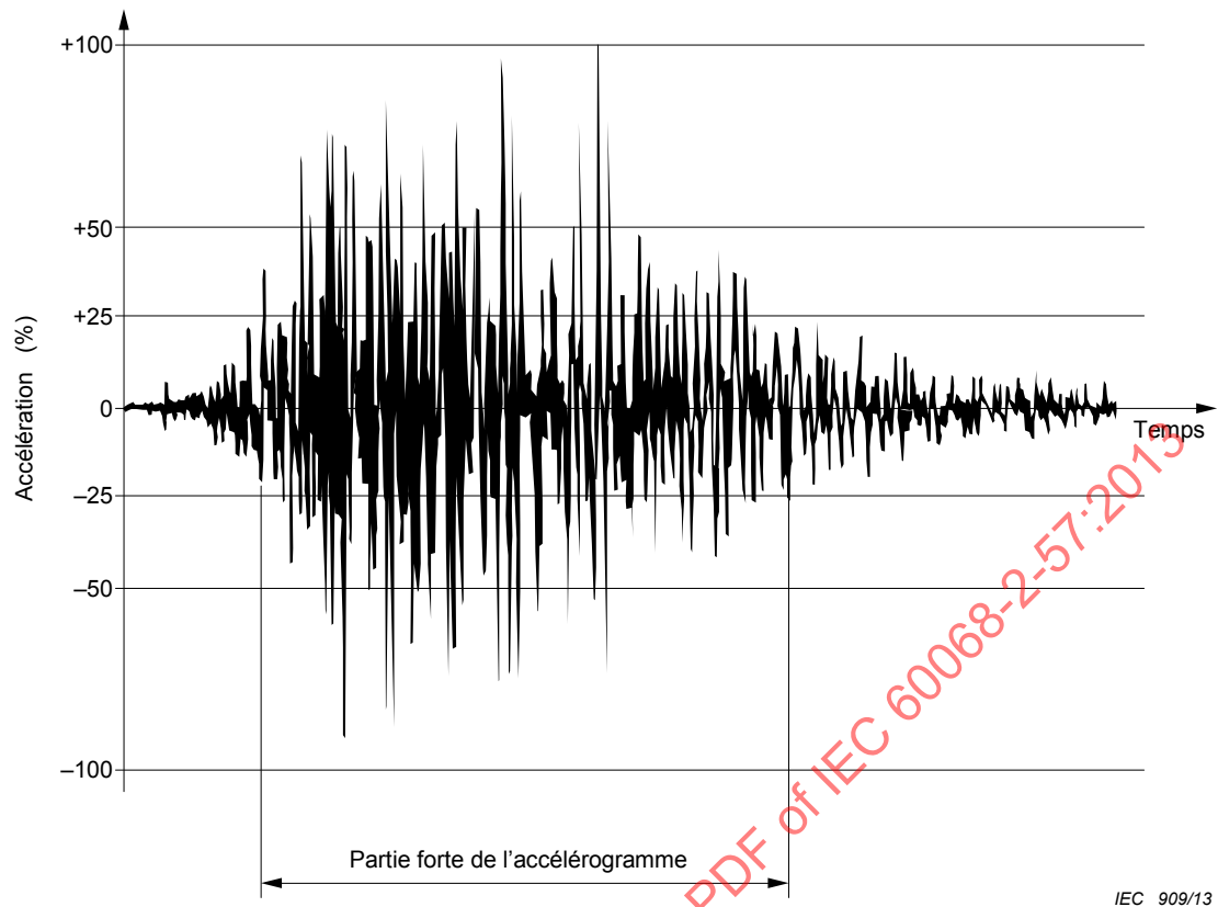
Figure 3 – Accélérogramme caractéristique
