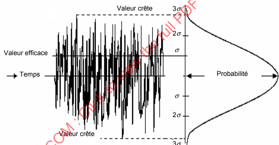
Figure 2 – Accélérogramme de l'excitation stochastique; fonction de la densité de probabilité avec distribution (normale) gaussienne (exemple avec le facteur de crête = 3, voir aussi 3.14 et 4.6.2)
