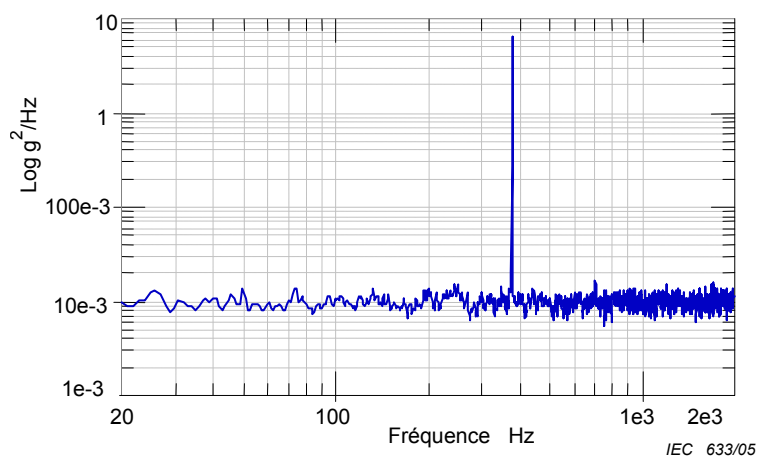
Figure A.2 – Sinus à 380 Hz
