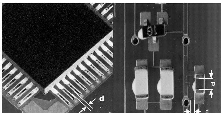
Figure D.1 – Plus petite distance des composants et des cartes de circuits imprimés
