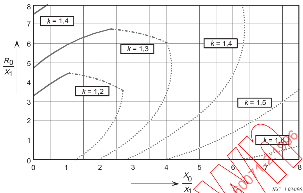
Figure B.5 – Relation entre R_0/X_1 et X_0/X_1 pour des valeurs constantes du facteur de défaut à la terre k lorsque R_1 = 2X_1
