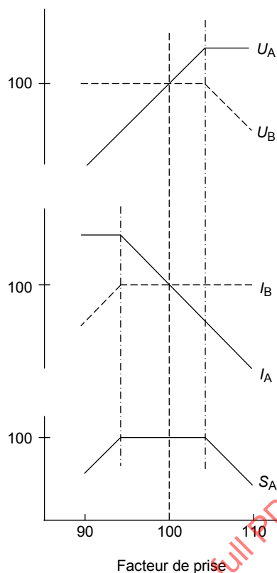
Figure 1c – Réglage combiné (RCb ou CbVV)
