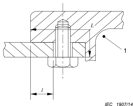
Figure 8 – Orifices aux surfaces des joints à emboîtement, exemple 3
