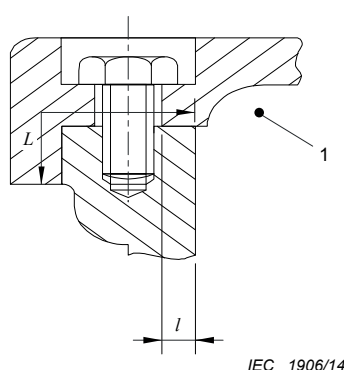
Figure 7 – Orifices aux surfaces des joints à emboîtement, exemple 2
