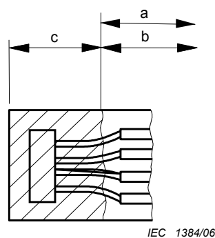
Figure 4a – Carte partiellement revêtue
