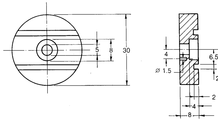
FIG. 2. — Disque-électrode en cadmium.
