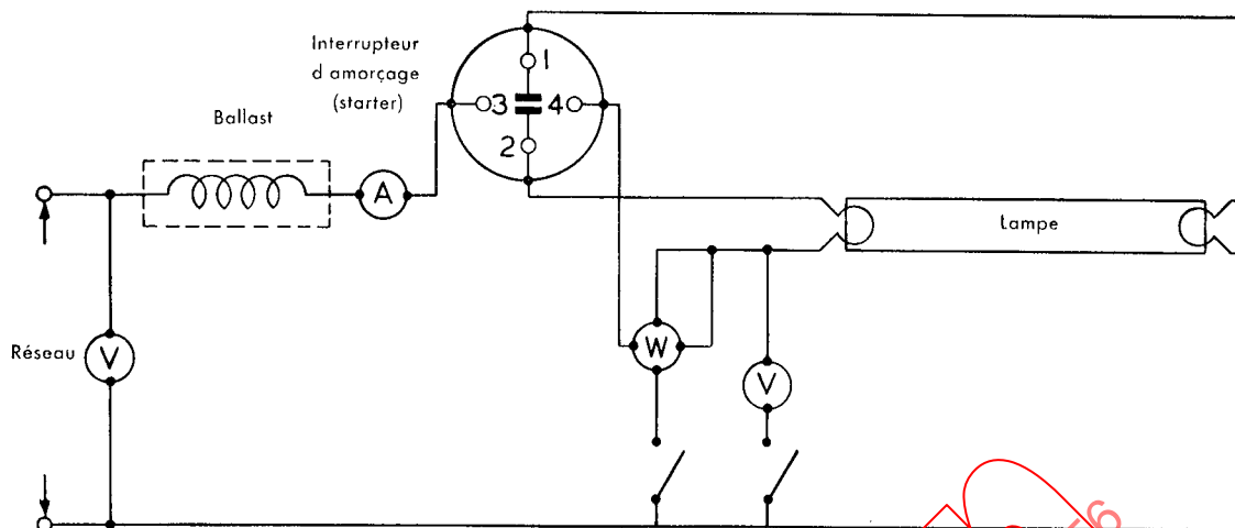
Figure 2 Circuit d'essai pour le relevé des caractéristiques
