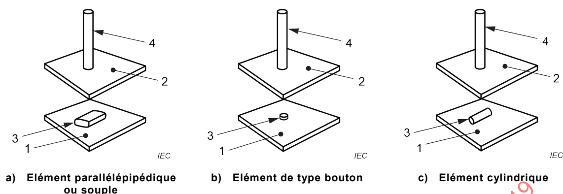
Figure 3 – Exemples de montage d'essai pour l'essai d'écrasement
