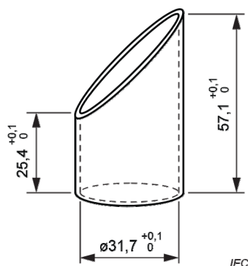
Figure 8 – Gabarit d'ingestion
