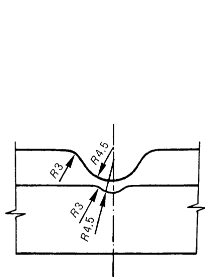
FIG. 3a. — Détail X — encoche. Detail X — notch.
