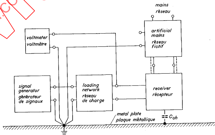
Fig. 3 (Clause 3.1.3) — Circuit arrangement for measurement of radiation via the mains. Fig. 3 (Article 3.1.3) — Montage pour la mesure des rayonnements par le réseau.
