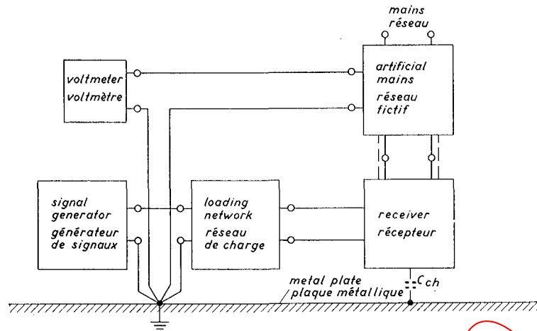
Fig. 1 (Clause 3.1.2) — Circuit arrangement for measurement of radiation via the aerial. Fig. 1 (Article 3.1.2) — Montage pour la mesure des rayonnements par l'antenne.
