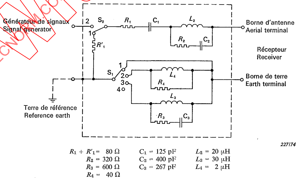
FIG. 2 (Article 4) — Réseau de charge.
