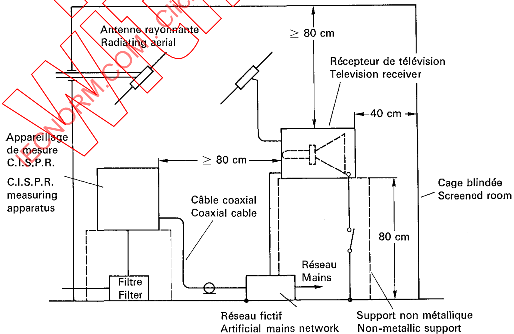
FIG. 8 (Article 18) — Mesure de la tension perturbatrice à radiofréquence injectée dans le réseau (Clause 18) — Measurement of the radio-frequency interference voltage injected into the mains.
