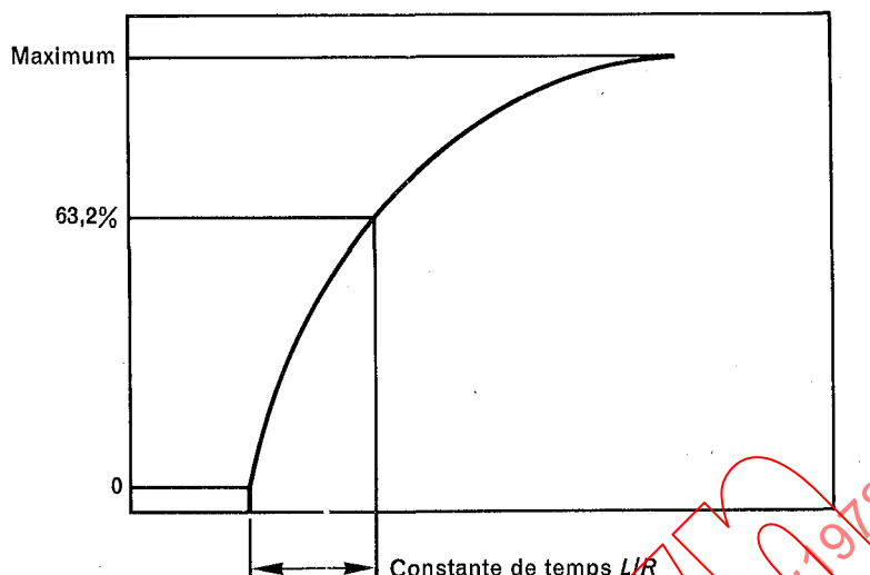
FIG. 2. — Oscillogramme.
