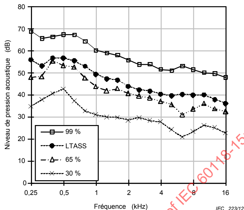
Figure 3 – 30°, 65°, 99° centiles de l'ISTS et niveaux de pression acoustique du LTASS en dB en fonction de bandes d'un tiers d'octave
