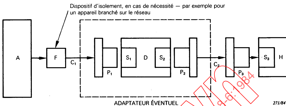
FIG. A1. — Exemple d'une disposition schématique du circuit reliant l'appareil de correction auditive à la source extérieure de signal.
