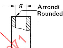
FIG. 16. — Douille. Socket.
