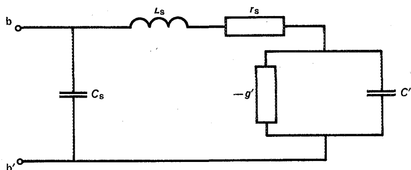
FIG. 5. — Circuit équivalent d'une diode tunnel.
