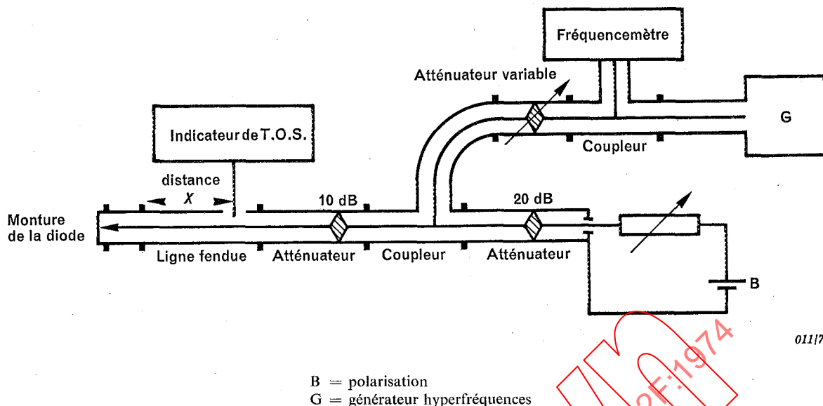
FIG. 9. — Montage pour la mesure de l'inductance série.
