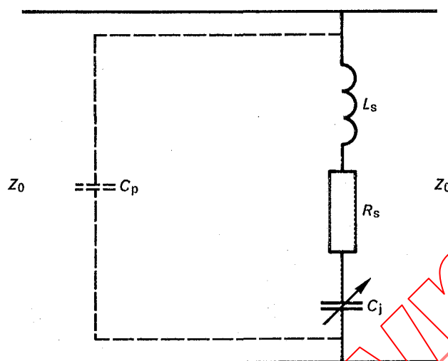
FIG. 24. — Circuit équivalent de la diode dans sa montage.
