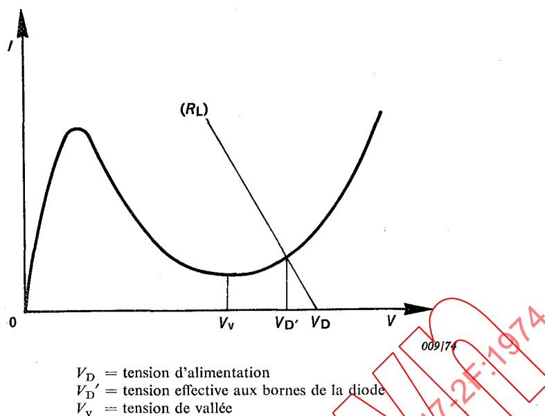
FIG. 7. — Caractéristique d'une diode tunnel comprenant la diode de charge.
