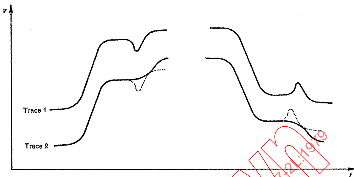
FIG. 8. — Traces non coïncidentes dues à une modification de l'équilibre à l'aide du circuit en mesure (les lignes pointillées montrent le rétablissement de l'équilibre au moyen de R_2 et C_2 ).
