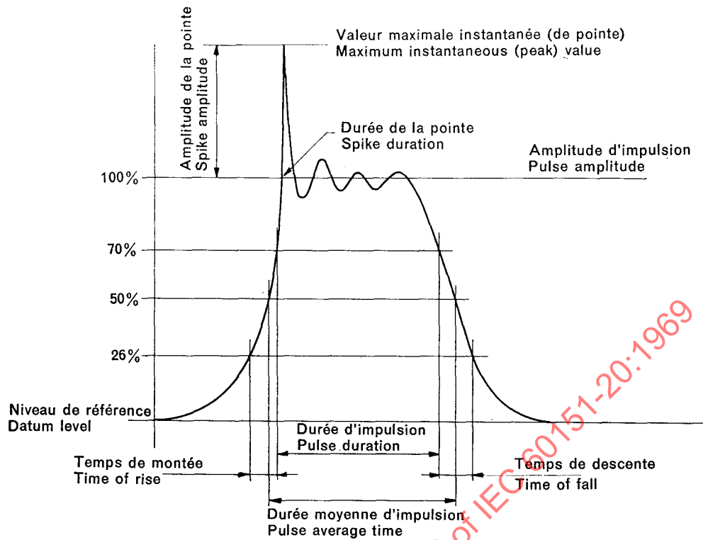
FIG. 1. — Caractéristiques de l'impulsion. Pulse characteristics.
